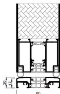
Seuil alu encastrable avec panneau
