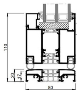
Seuil alu encastrable avec vitrage
