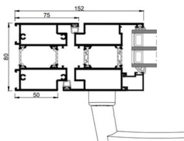
Porte pivot avec vitrage
