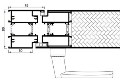
Porte pivot avec panneau monobloc
