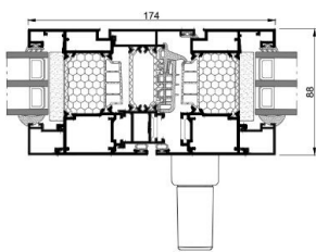
Battement 2 vantaux
