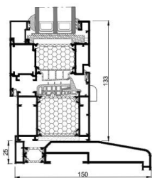
Ouvrant avec pièce d'appui
