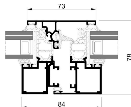
Coupe 70 HO 2 OB battant central
