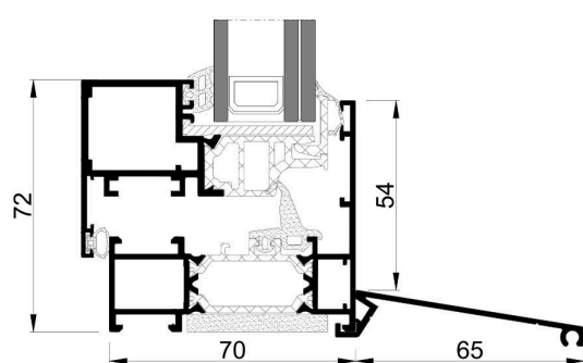
Coupe 70 HO avec bavette
