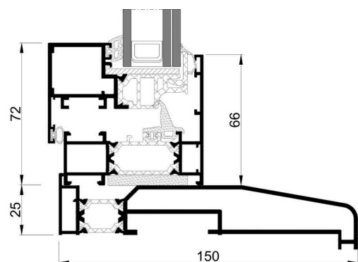
Coupe 70 HO avec pièce d'appui
