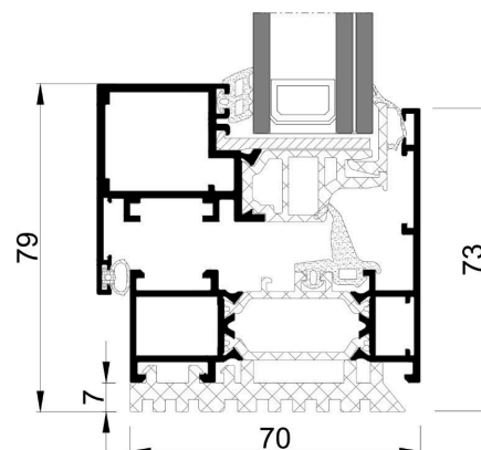
Coupe 70 HO avec drainage caché
